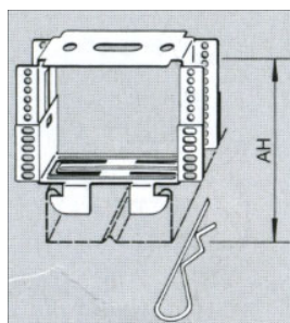
Direktabhänger justierbar
