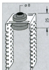
Direktabhänger Schallschutz
