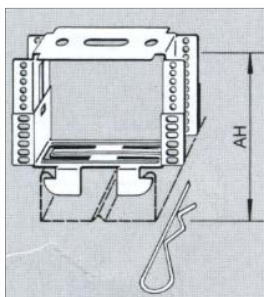
Direktabhänger Justierbar
