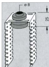
Direktabhänger Schallschutz
