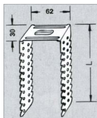
Direktabhänger Normal
